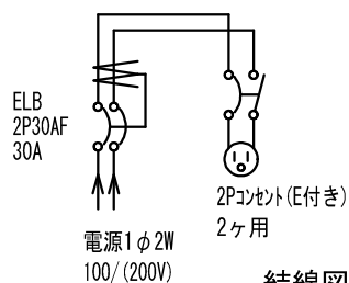
結線図
